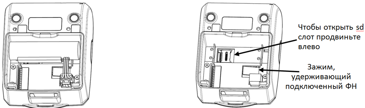
Рис.1 Внутренний отсек ККТ
